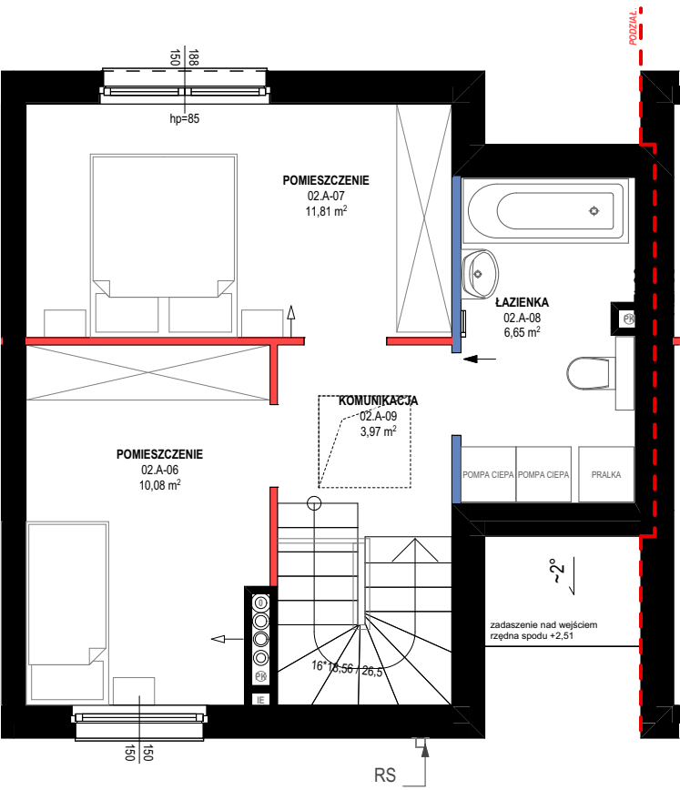
RZUT 1 PIĘTRA
