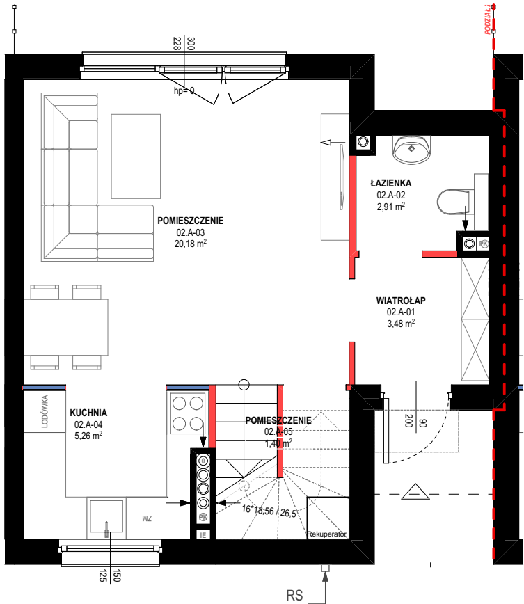
RZUT PARTERU
